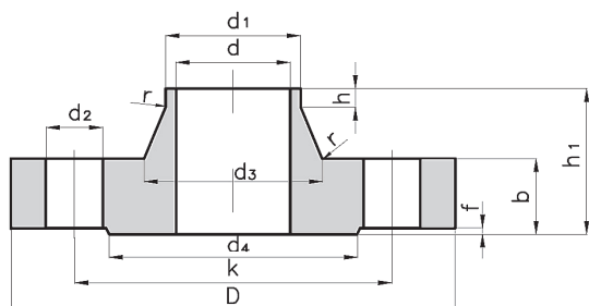
d 4 hladká těsnicí lišta
