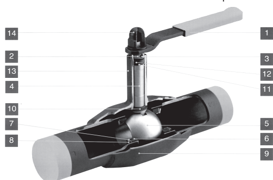
ovládání pákou
