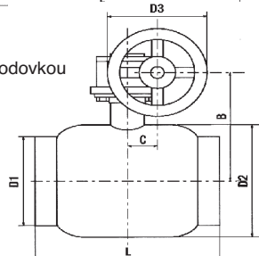
Rozměrová tabulka
