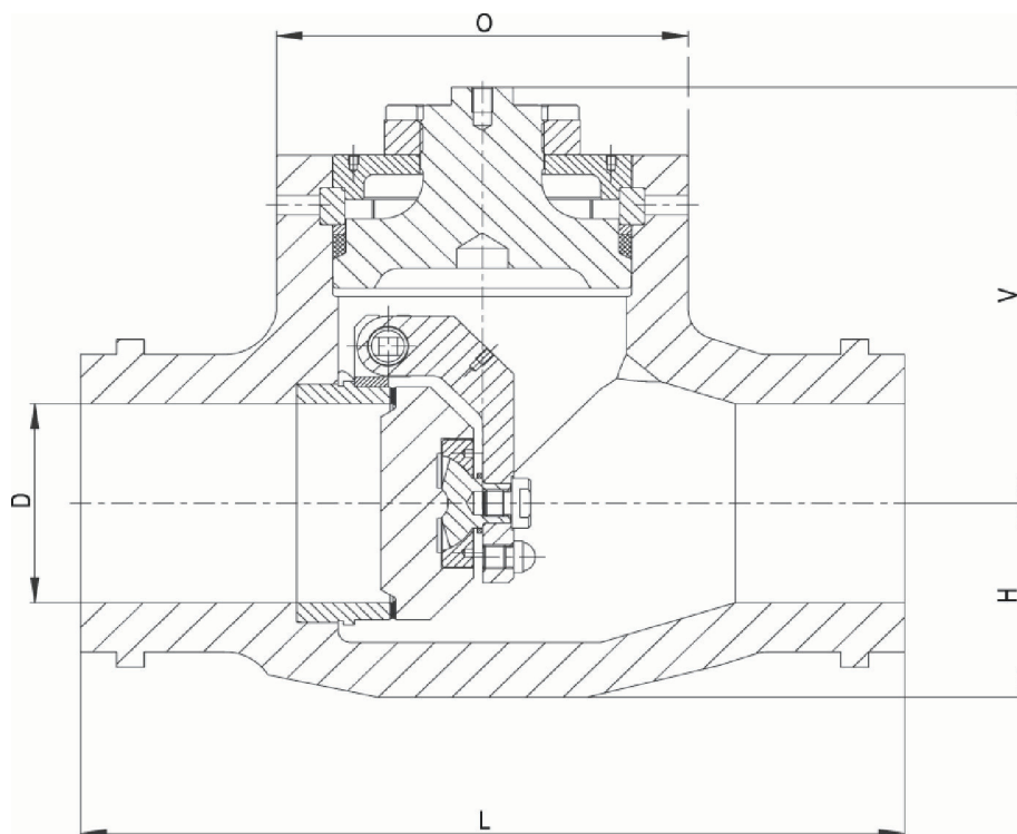
Tabulka stavebních rozměrů - PN 63 - 400
